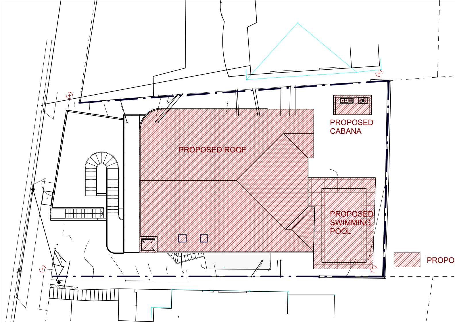
1 NP - SITE PLAN DA17 1 : 200
